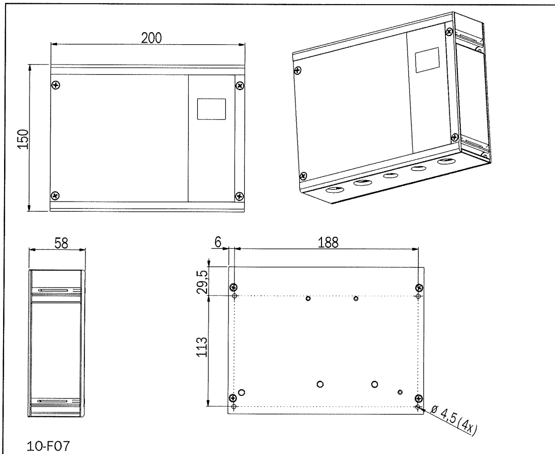
Abb. 8 Abmessungen - Steuergerät (mm)
